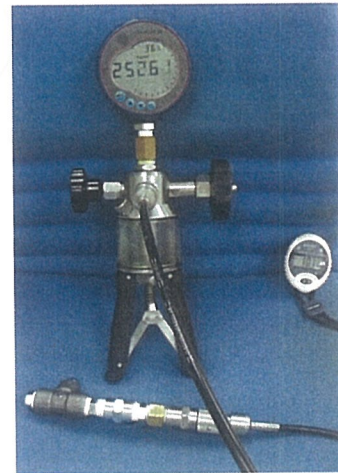
耐水壓試驗
