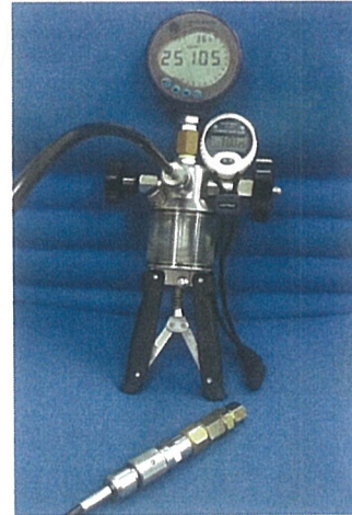
耐水壓試驗
